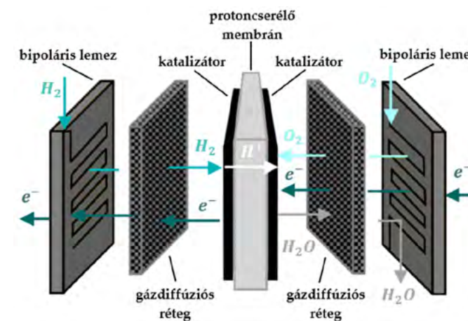
△ 1. ábra: A hidrogén-cella felépítése [4]
