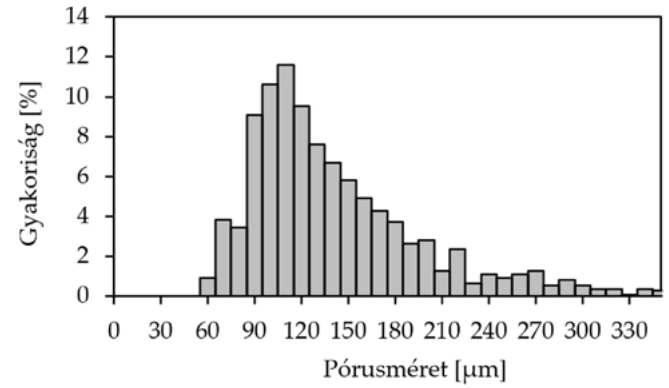
△ 5. ábra: A hab pórusméreteloszlása
