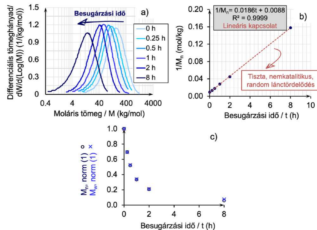
△ 2. ábra: A molekulatömeg változása a besugárzási idő függvényében: a) a besugárzott PLA minták molekulatömeg-eloszlása, b) a szám szerinti átlagos molekulatömeg és a besugárzási idő inverze közötti kapcsolat, c) normalizált szám- és tömeg szerinti átlagos molekulatömeg.
