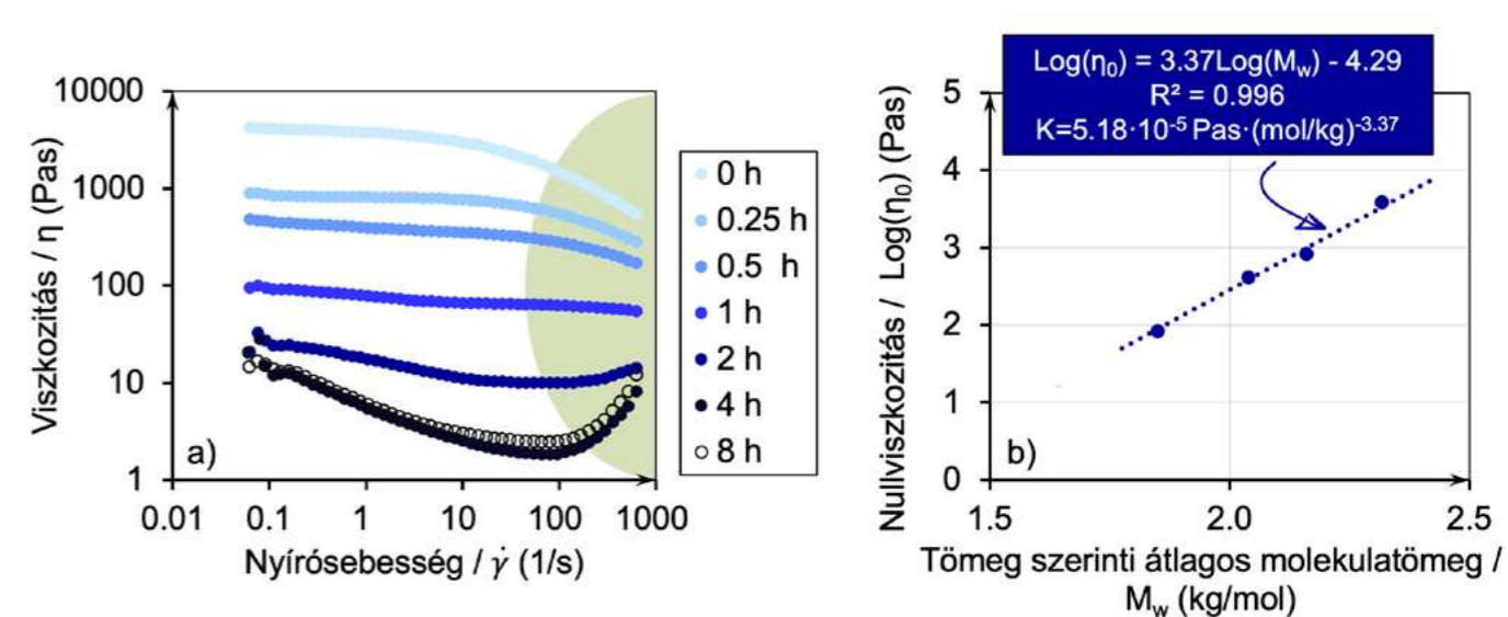
4. ábra: UV-C besugárzás hatása a viszkozításra: a) nyírsebességfüggő viszkozitás, b) nullviszkozitás a tömeg szerinti átlagos molekulatömeg függvényében
