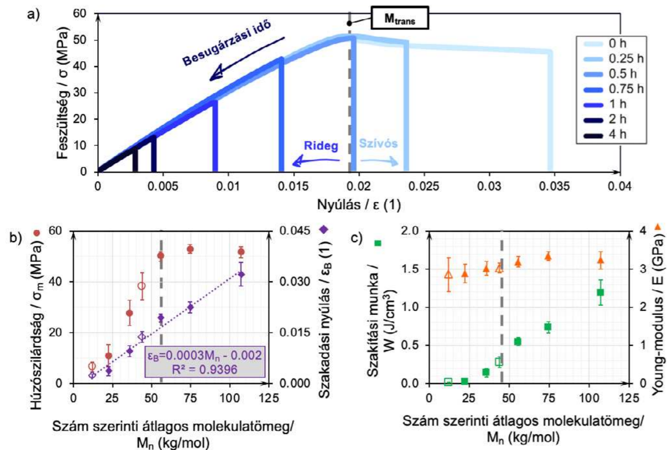
3. ábra: a) A szakítógörbe alakjának változása a besugárzás hatására. b) A húzószilárdság és a szakadási nyúlás alakulása a tömeg szerinti átlagos molekulatömeg függvényében. c) A szakítási munka és a Young-modulus alakulása a szám szerinti átlagos molekulatömeg függvényében. A teli körök a mért molekulatömegekhez tartozó tulajdonságok, az üres körök a lineáris regresszióból becsült molekulatömegekhez tartozó mért tulajdonságok. Az illesztéshez csak a teli körrel jelölt adatokat használtuk.
