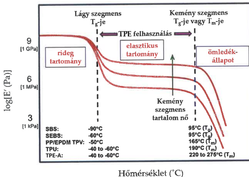
1. ábra: Tárolási modulusz a hőmérséklet függvényében, húzó elrendezésből kapott dinamikus mechanikai analizisből. SBS: sztírol-butadién-sztírol; SEBS: sztírol-etilén-butilén-sztírol; PP/EPDM: polipropilén/etilén-propilén-dién monomer; TPU: termoplasztikus poliuretán; TPE-A: amid alapú termoplasztikus elasztomer. Jelleghelyes ábra TPE-k esetében [11]
